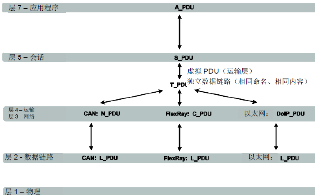
图A.1 任一通信协议的 T_PDU 虚拟 PDU 接口
